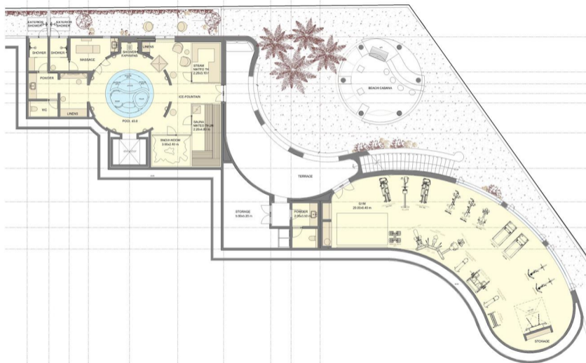
NIVEL SOTANO SPA & GYM
